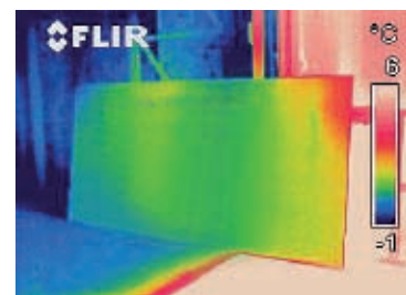
Air Door ausgeschaltet
