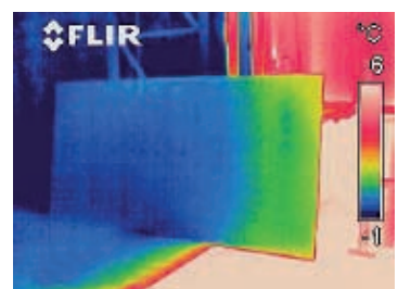
Air Door eingeschaltet
